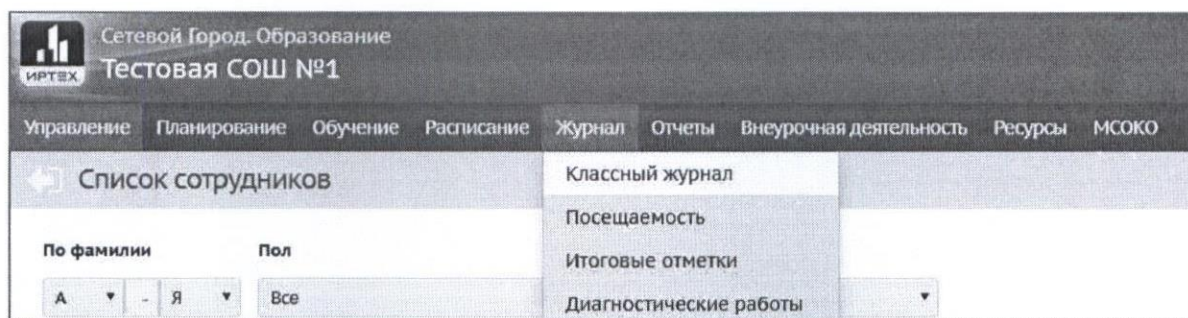
Рисунок 1 – Функция «Журнал»
