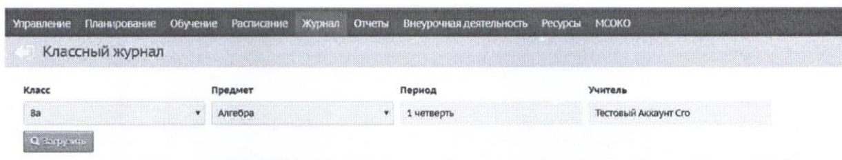
Рисунок 2 – Классный журнал
